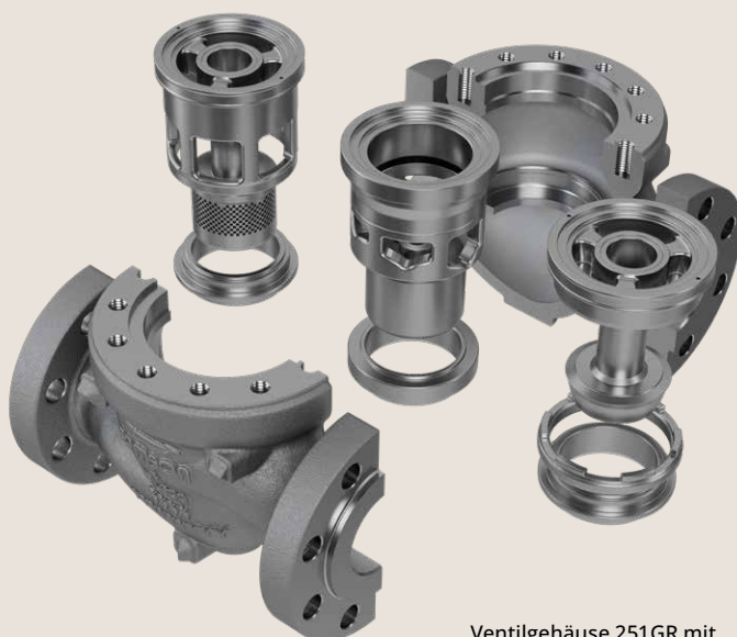
Ventilgehäuse 251GR mit verschiedenen Regelgarnituren
