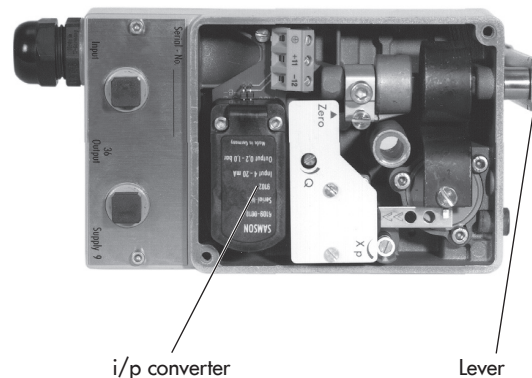
Fig. 3: Type 4763 Positioner
