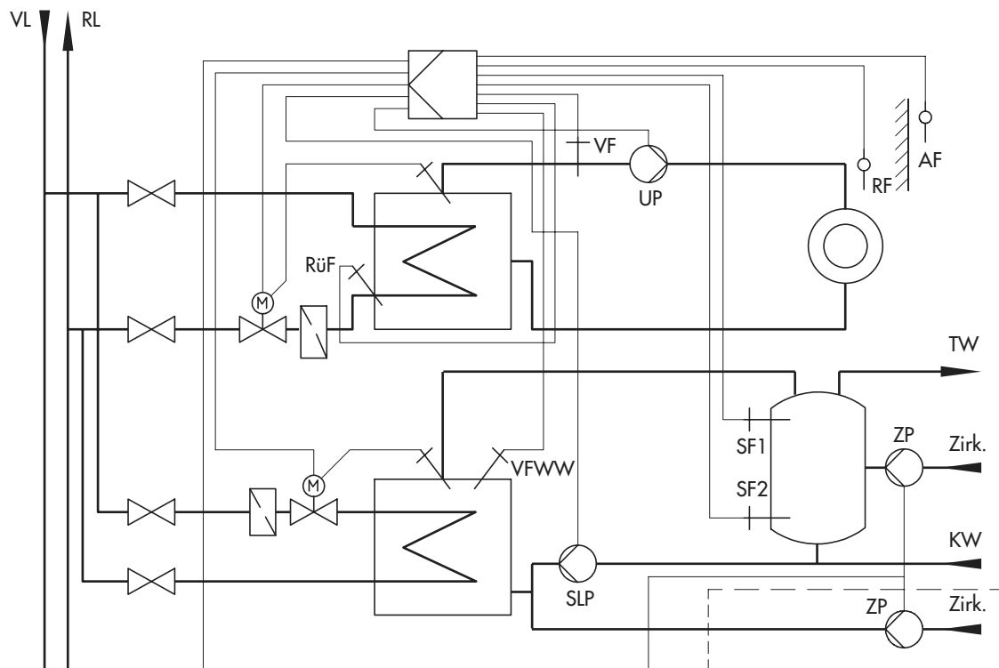
Rys. 8 · Schemat instalacji 5.0
