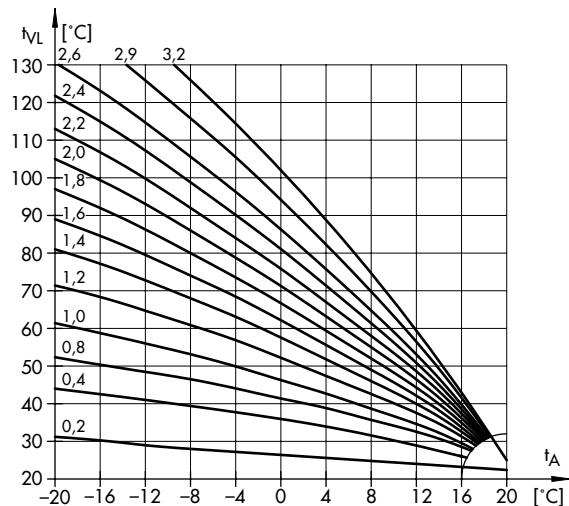
Rys. 4 · Krzywe grzania
