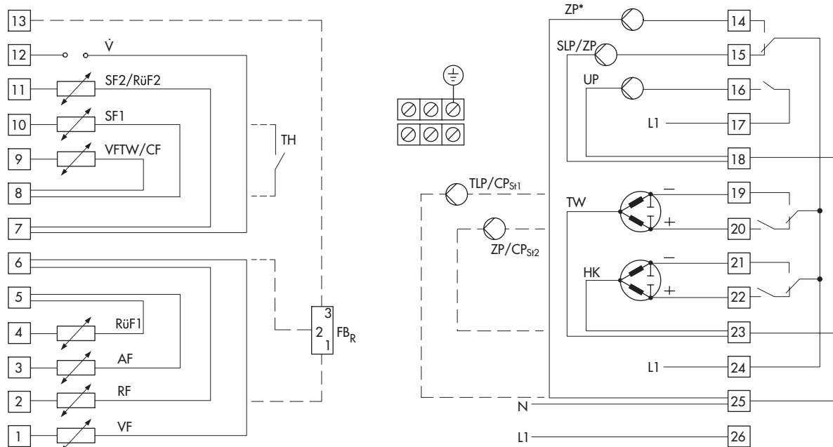
Rys. 9 · Przyporządkowanie zacisków
