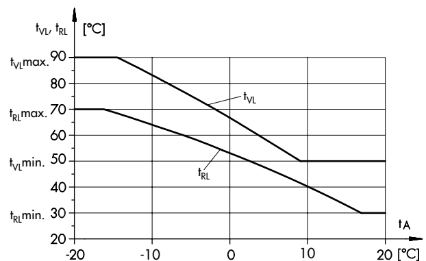
Rys. 5 · Pogodowa regulacja temperatury zasilania z płynnym ograniczeniem temperatury powrotu
