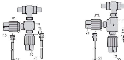
Temperaturregler mit Doppelanschluss Do3 Temperaturregler mit Sicherheitstemperaturbegrenzer (STB)
