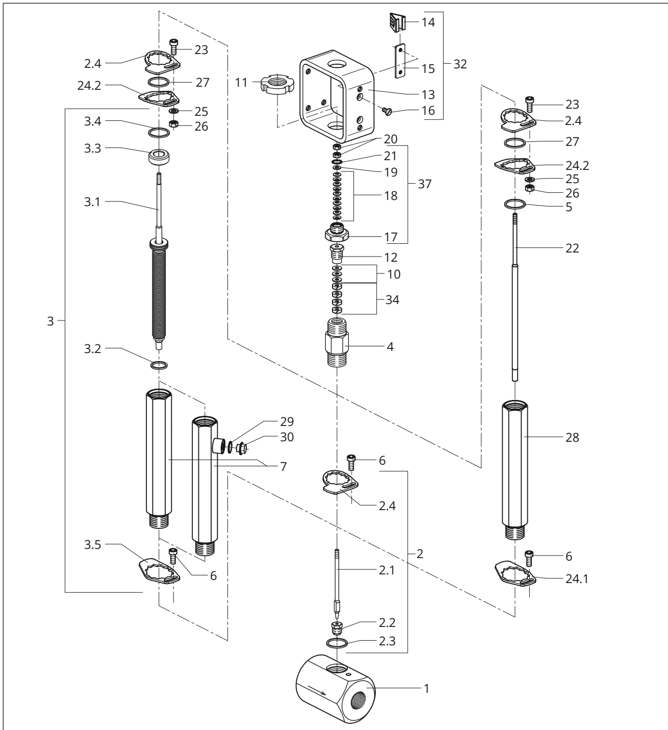
Bild 1: Mikroventil Typ 3510 · Explosionszeichnung
