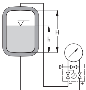
Schema 1 Messung bei Tiefkälteanlagen (verflüssigte Gase)
