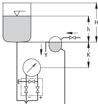
Schema 3 Messung an offenen Behältern bei tiefliegendem Messgerät
