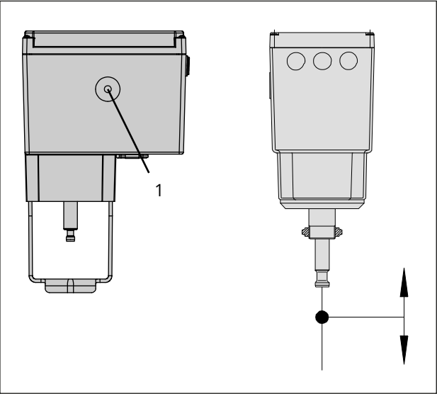
Bild 52: Mechanische Handverstellung
