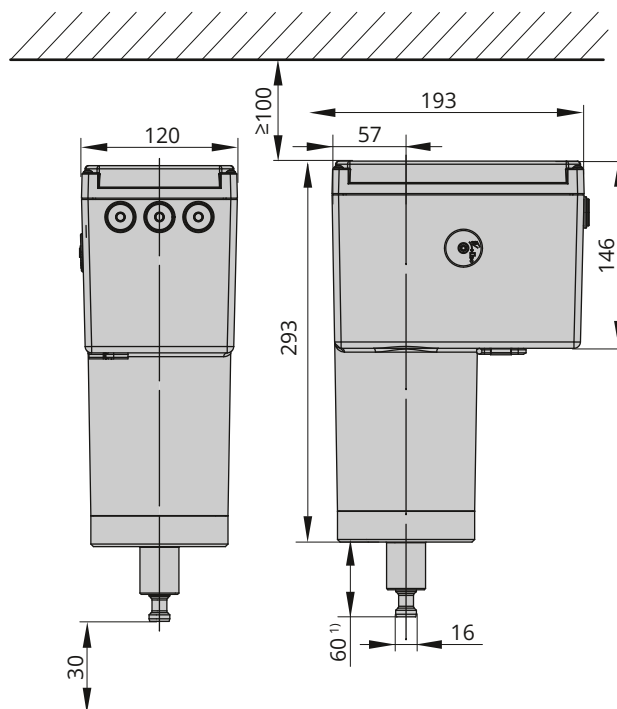
Bild 7: Maße in mm · Typ 3374-35, Ausführung Form A
