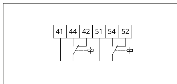
Bild 34: Elektronische Grenzkontakte
