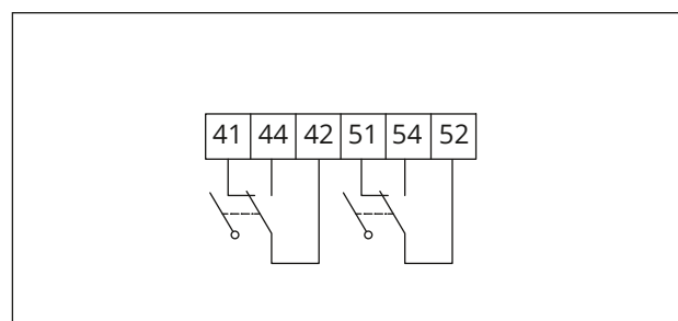
Bild 33: Mechanische Grenzkontakte
