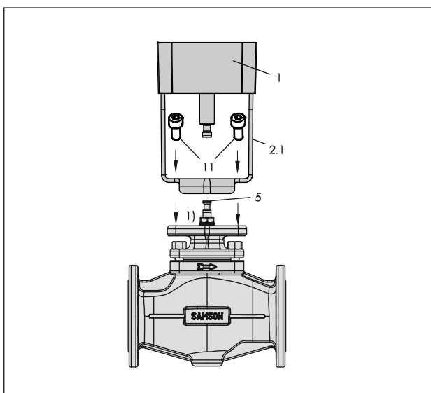
Bild 13: Anbau · Ausführung mit Antriebsjoch und Zubehör V2001
