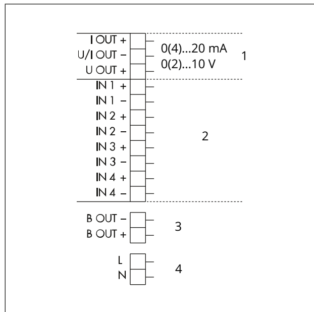
Bild 25: Elektrischer Anschluss
