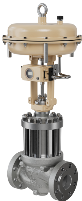
Pneumatisches Stellventil SMS HG-1: Ventil Typ 261GR mit Antrieb Typ 3271
