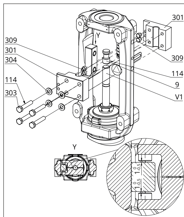
Bild 15: Montageübersicht der Verdrehsicherung in der Sonderausführung
