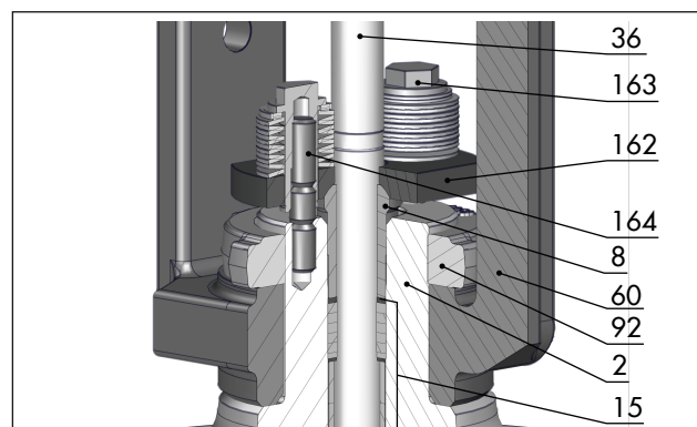
Bild 21: Packung mit außen federbelasteter Packungsbrille
