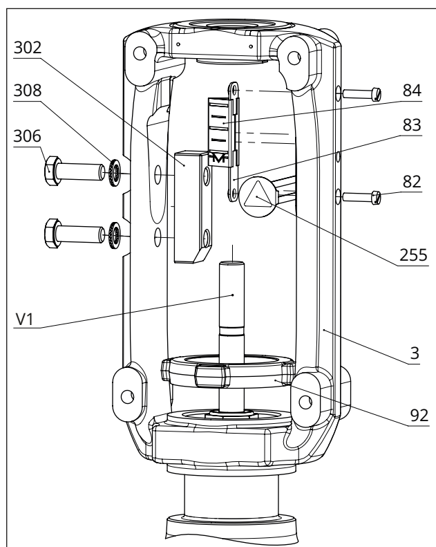
Bild 14: Montageübersicht der Baugruppe Joch mit Hubschild in der Sonderausführung
