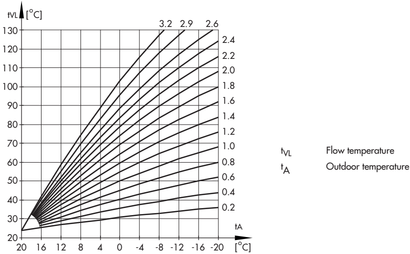
Fig. 5 · Gradient characteristics
