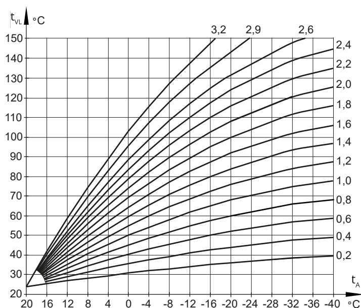
Bild 11: Steigungskennlinien
